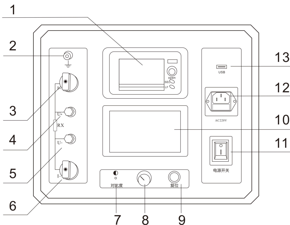
图 1 面板结构图
